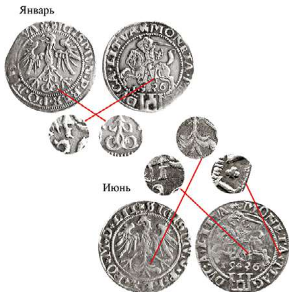
Отличия грошей с буквой І «январской» и «июньской» чеканок Рисунок 18
